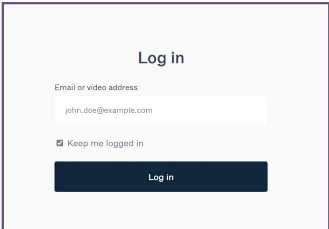
Afbeelding 4: inlogscherm Pexip
