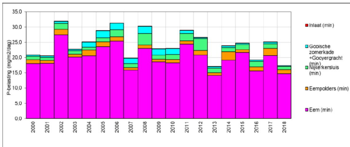
Figuur 10 Berekende fosfaat-belasting (mg/m 2 /dag) op jaarbasis opgesplitst per bron voor het Eemmeer
