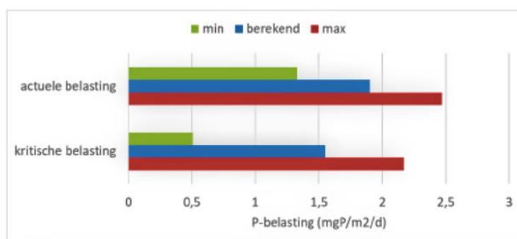
Figuur 5 Actuele en kritische fosfaatbelasting met onzekerheidsmarges 40% voor de kritische belasting en 30% voor de actuele belasting
