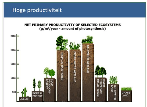
Figuur 12 Organische productie in diverse ecosystemen
