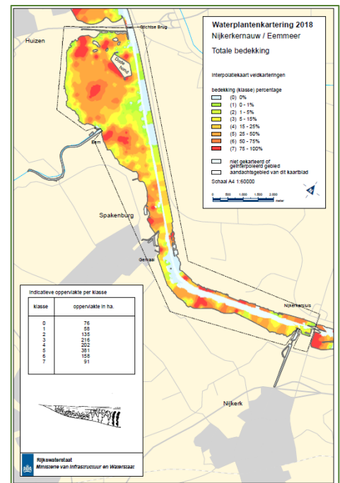
Figuur 22 Totale waterplanten bedekking Eemmeer/Nijkerkernauw 2018
