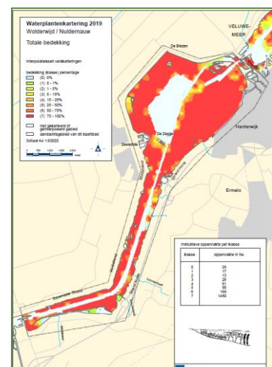
Figuur 21 Totale bedekking waterplanten Wolderwijd en Nuldernaau 2019
